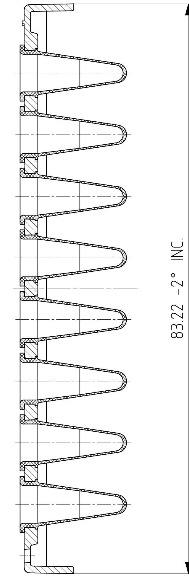
SECTION A-A
