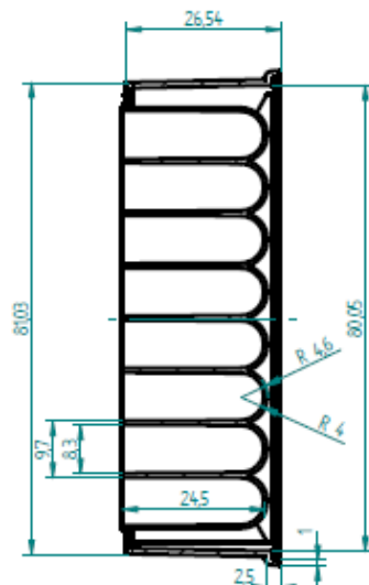
Schnitt X-X
