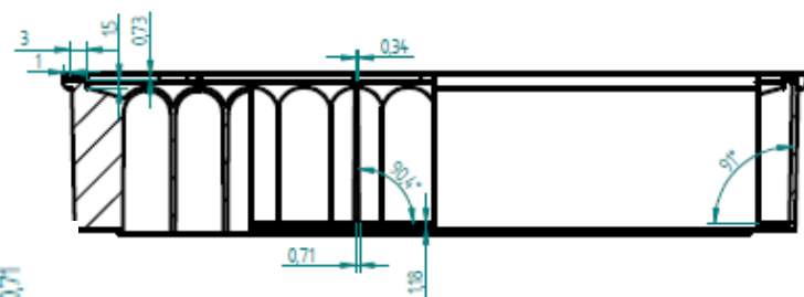
Schnitt Y-Y
