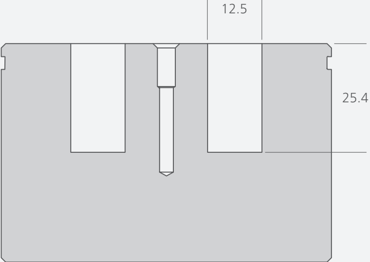
A-A (1:1)
